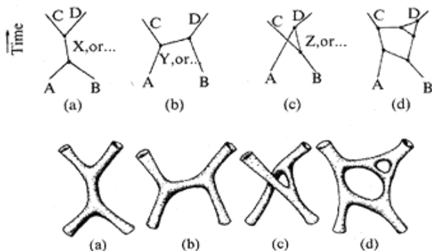
شکل ۱۴ - دیاگرامهای فینمن در تئوری ذرات نقطه‌ای (بالا) و تئوری رشته‌ها (پائین).
