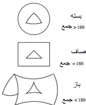
شکل ۶ - از بالا به پائین، جهان بسته، جهان مسطح و جهان باز.
