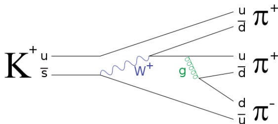
شکل ۱۳ - دیاگرام فینمن که در آن یک ذره‌ی کائون K با واپاشی ضعیف و قوی به سه عدد پیون تبدیل می‌شود. چنانکه می‌بینیم در مسیر این واپاشی پله‌هانی هستند که در آن بوزون W و گلئون g نیز تولید شده‌اند.
