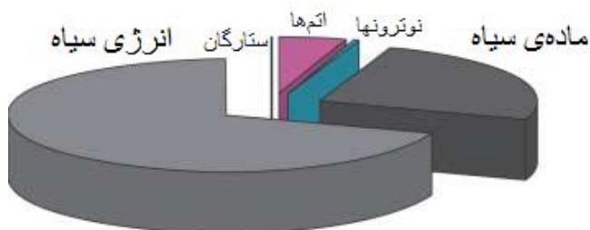
شکل ۱۰ مقدار محاسبه شده‌ی اجزاء تشکیل دهنده‌ی جهان!
