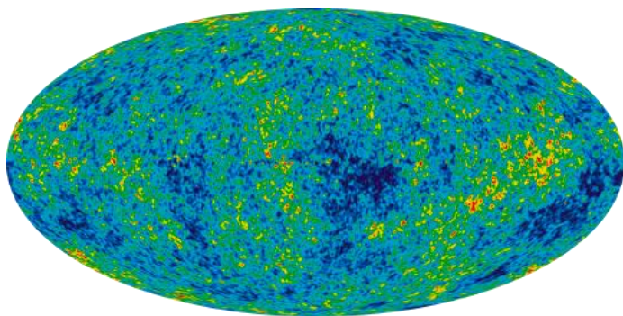
شکل ۸ - رنگها ساختگی هستند ولی هر رنگی نشان‌دهنده‌ی یک طول موج خاصی است. این تصویر نشان می‌دهد که جهان همگن نیست بلکه دارای پستی و بلندی است.
