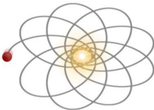
شکل ۳ مدار چرخش عطارد بر گرد خورشید
